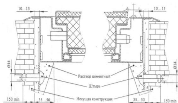
Рис.1 Схема монтажа Блока дверного
